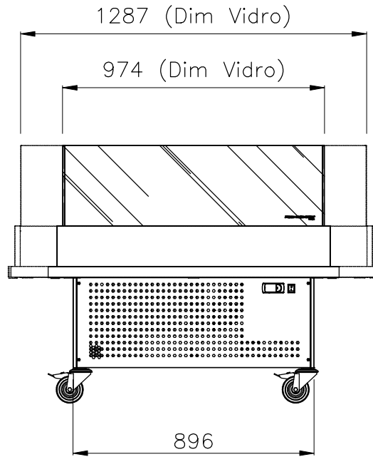
Escala / Écaille / Scale / Escala / Scala: 1/20
