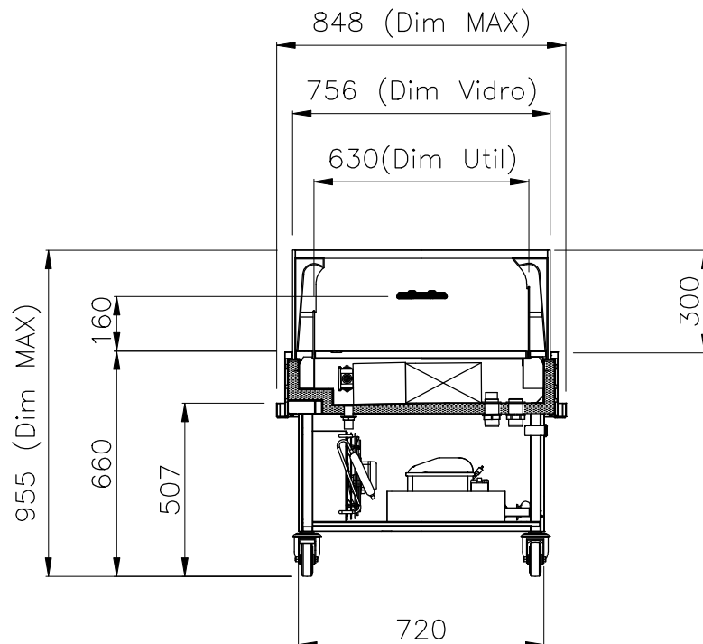
Escala / Écaille / Scale / Escala / Scala: 1/20
