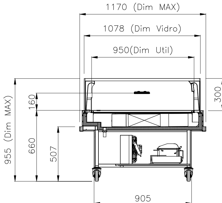
Escala / Échelle / Scale / Escala / Scala: 1/20
